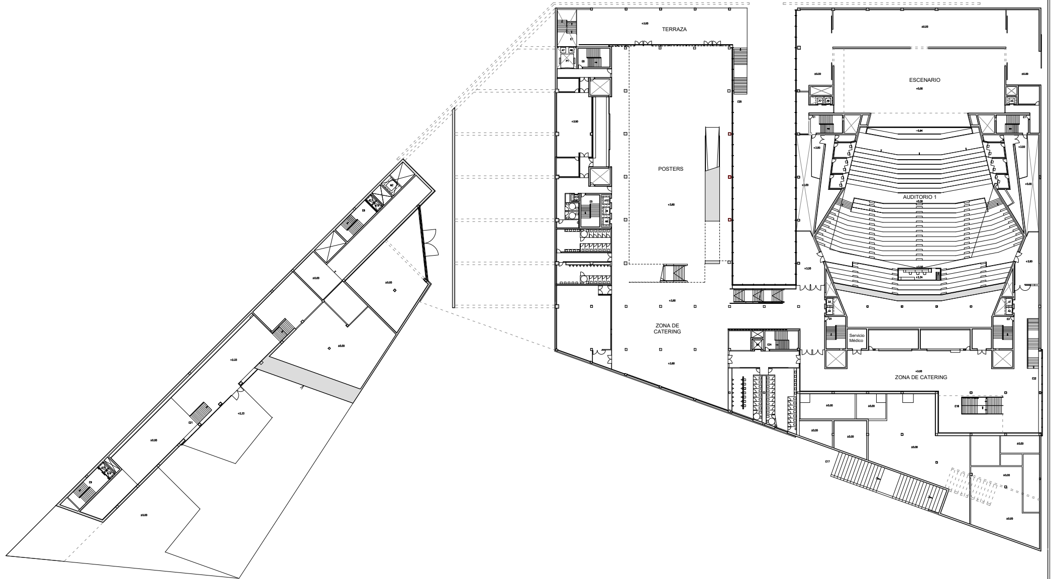
PLANO GENERAL FIBES II Planta 1 (Cota +3.50)
